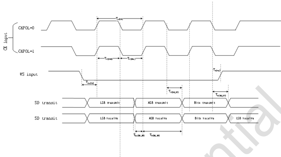
图 5-6 I 2 S 从模式时序图 (Philips 协议)
